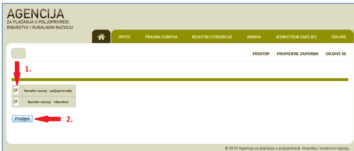
Slika 38. Pridjeljivanje modula
